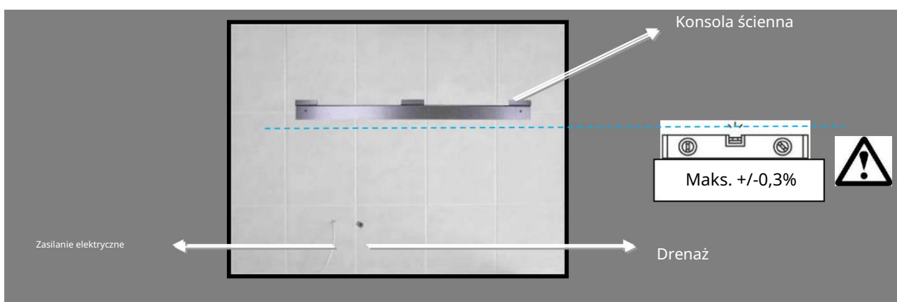
Przygotowanie zasilania elektrycznego, odpływu kondensatu i montażu konsoli
