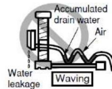
Nieprawidłowy montaż węży kondensatu
