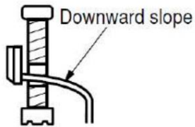
Prawidłowy montaż węży kondensatu
